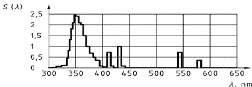
Рисунок В.1 – Спектральное распределение лампы
