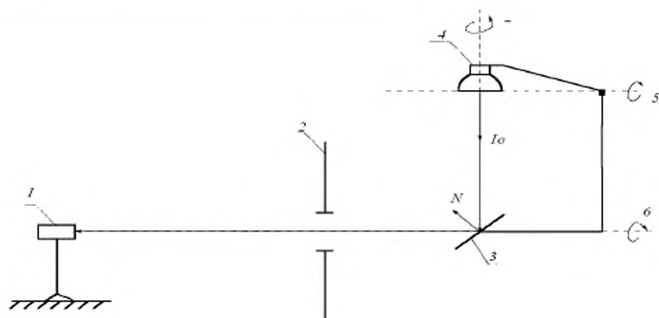
1 – фотометрическая головка; 2 – экран; 3 – зеркало; 4 – ОП; 5 – угол поворота \gamma ОП; 6 – угол поворота зеркала; 7 – ось вращения плоскостей в системе фотометрирования ( C-\gamma ); N – нормаль; I_0 – осевая сила света
