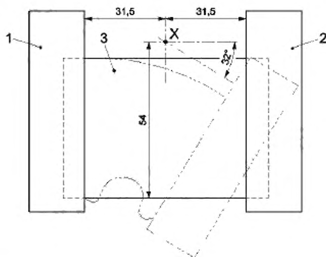
f — неподвижный зажим; 2 — движущийся зажим; 3 — образец для испытаний; X — точка вращения
