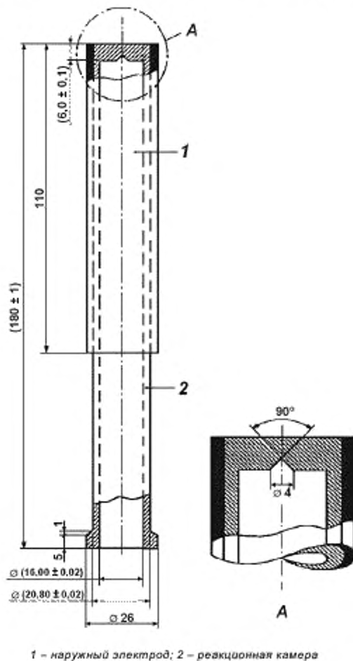
Рисунок 4 – Реакционная камера
