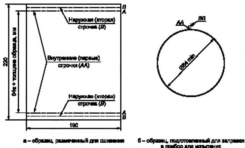
Рисунок 1.4 — Форма образца для испытания на скручивание/изгиб
