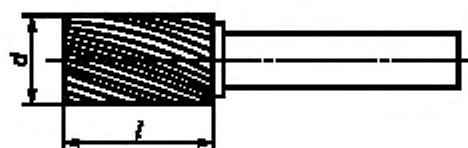
Рисунок 1 — Борфрезы типа А
