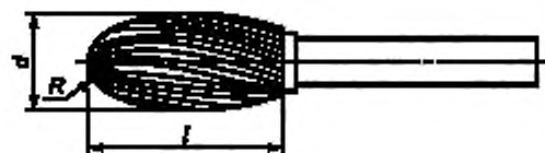
Рисунок 4 — Борфрезы типа E
