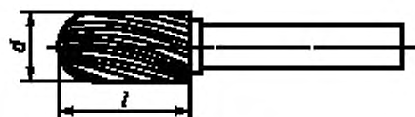
Рисунок 2 — Борфрезы типа С
