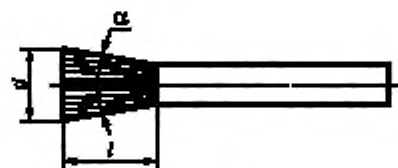
Рисунок 11 — Борфрезы типа N
