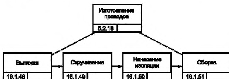
Рисунок В.6 — Процесс изготовления проводов изделия GT-350
