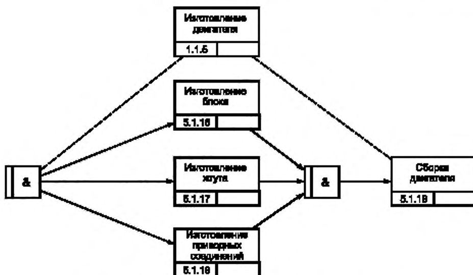
Рисунок В.2 — Процесс изготовления двигателя изделия GT-350
