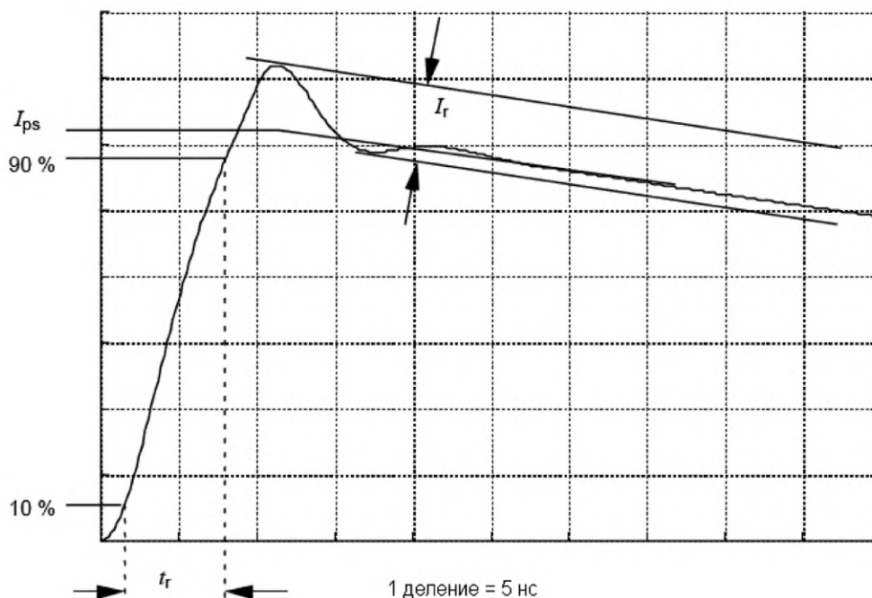
Рисунок 2а — Типичный импульс тока через закорачивающий провод t_g
