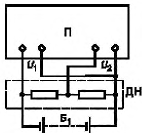
ДН — делитель напряжения, П — потенциометр постоянного тока, Б 1 — источник питания, U_1 и U_2 — измеренные значения входного и выходного напряжений делителя соответственно
