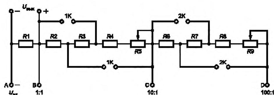
U_{\text{вх}} — входное напряжение; U_{\text{вых}} — выходное напряжение; A, B, C, D — клеммы подключения; R1-R4, R6-R8 — резисторы постоянные; R5, R9 — резисторы подстройки; 1K, 2K — контакты перемычек
