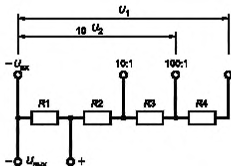
U_1 и U_2 — измеренные значения входного и выходного напряжений делителя соответственно; R_1, R_2, R_3, R_4 — сопротивления делителя
