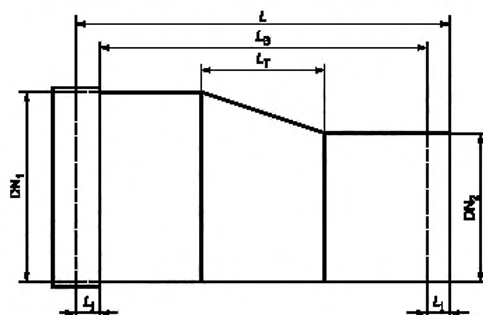
б — Переходник с эксцентричным расположением концевых отверстий
