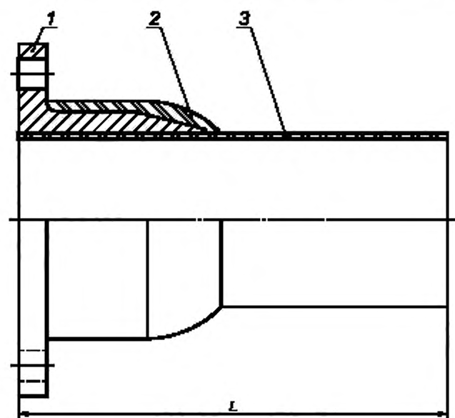
1 — фланец; 2 — полное обматывание из стеклопластика; 3 — раструб; L — длина переходника
