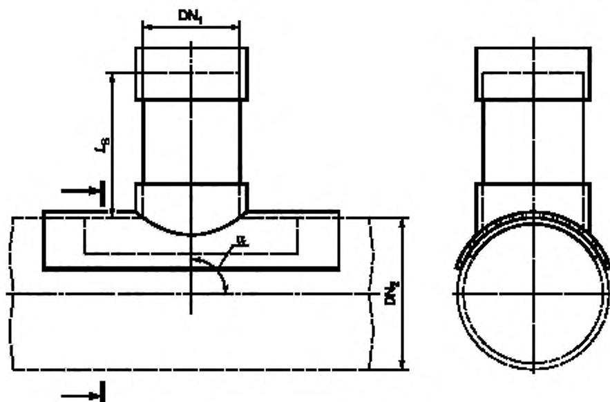
DN 1 — номинальный диаметр отводной трубы; DN 2 — номинальный диаметр главной трубы; L B — длина отводной трубы; α — установочный угол
