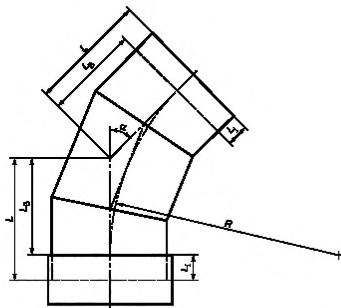
Рисунок 2 — Пример литого отвода
