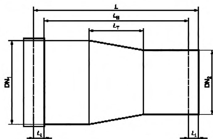
а — Переходник с концентричным расположением концевых отверстий
