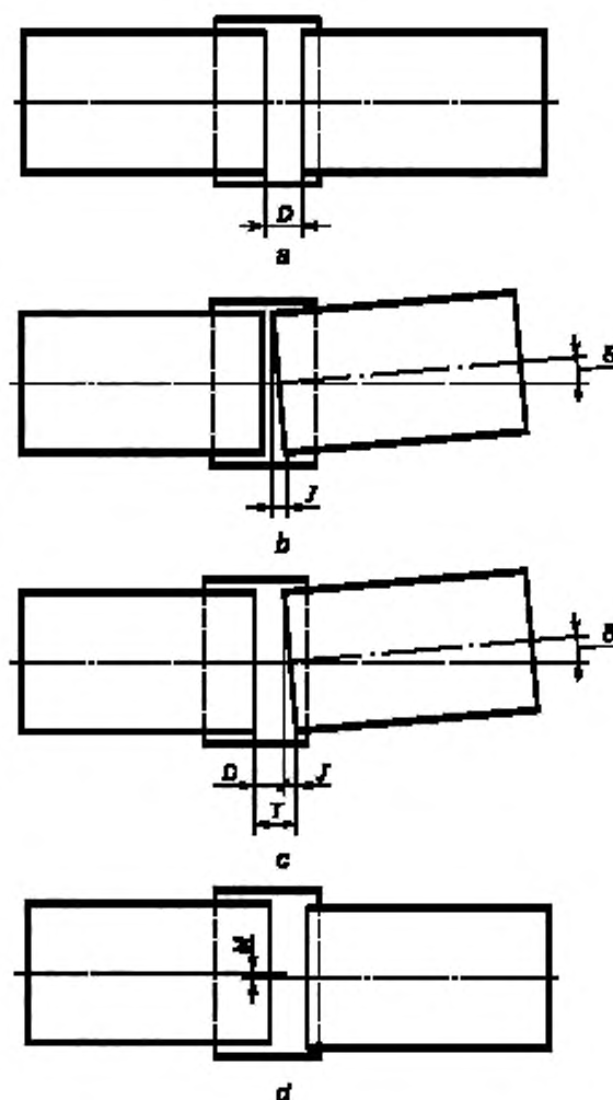
D — расхождение стыка; J — продольное смещение, возникающее из-за углового отклонения соединения; \delta — угловое отклонение соединения; T — общее расхождение стыка; M — осевое смещение.
