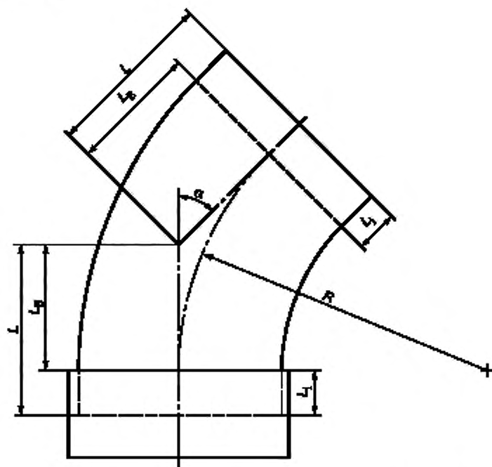
Рисунок 2 — Пример литого отвода
