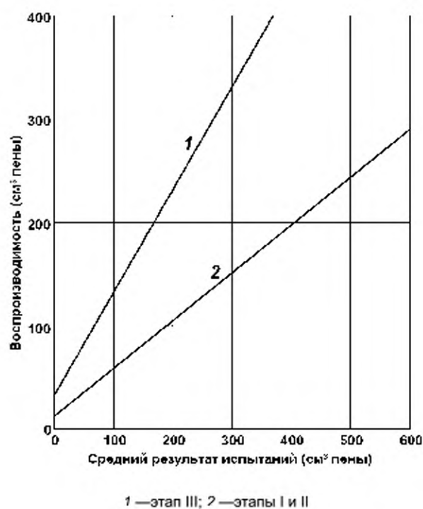
Рисунок 4 — Воспроизводимость
