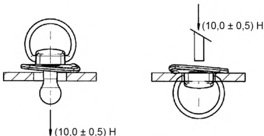
Рисунок 11 – Испытание защитного диска (5.2.3.2)
