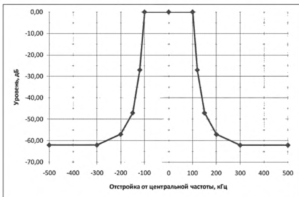
Рисунок 2 — Маска огибающей внеполосных радиоколечаний для ширины полосы частот 200 кГц
