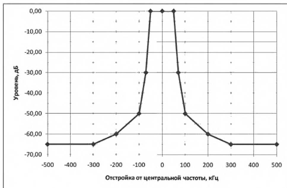
Рисунок 1 — Маска огибающей внеполосных радиоколечаний для ширины полосы частот 100 кГц
