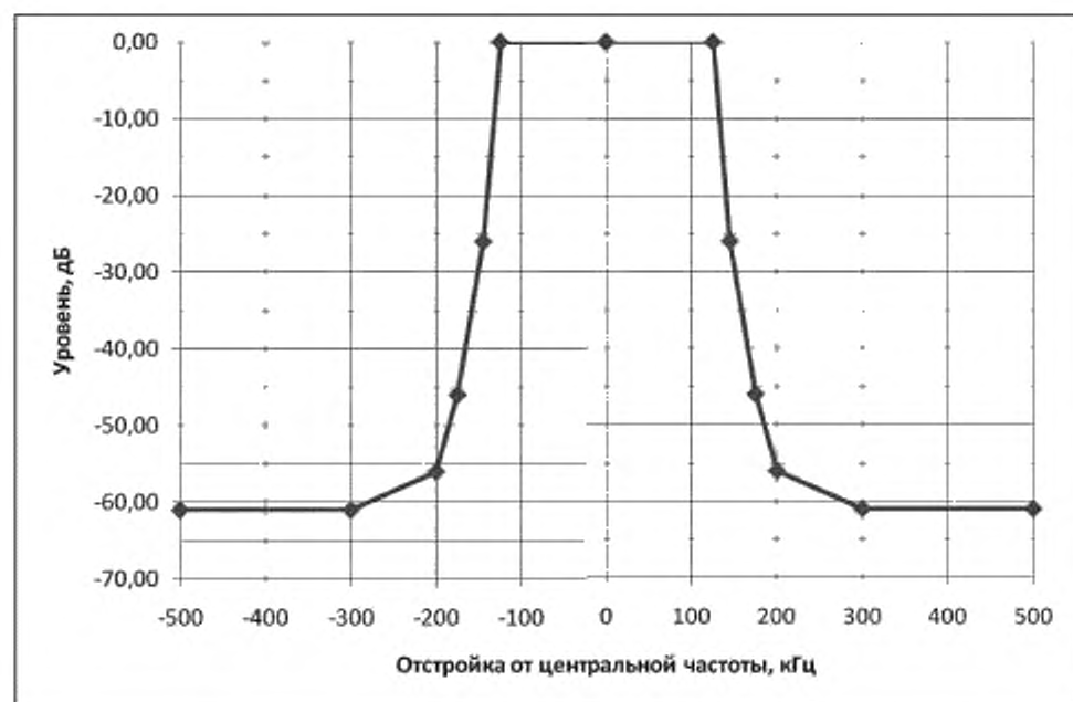
Рисунок 3 — Маска огибающей внеполосных радиоколебаний для ширины полосы частот 250 кГц
