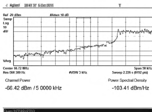
Рисунок В.26 – Плотность мощности минус 103,4 дБм/Гц на частоте f_{(0-115)}
