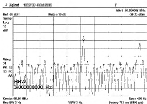
Рисунок В.38 – Полоса сканирования (Span) 400 Гц
