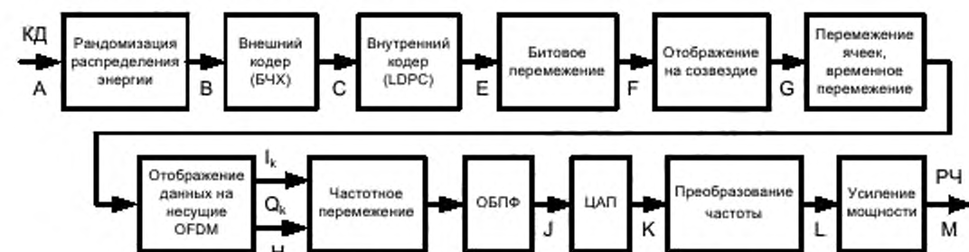
Рисунок 1 – Функциональная схема передающей части системы РАВИС (передатчик)
