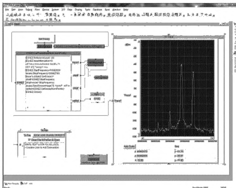
Рисунок В.6 – VEE Pro. Результаты измерений частот f_{(276)} и f_{(276), 20} и их разности
