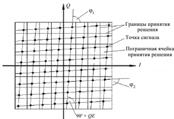
Рисунок 8 – Искажение диаграммы созвездия, вызванное квадратурной ошибкой
