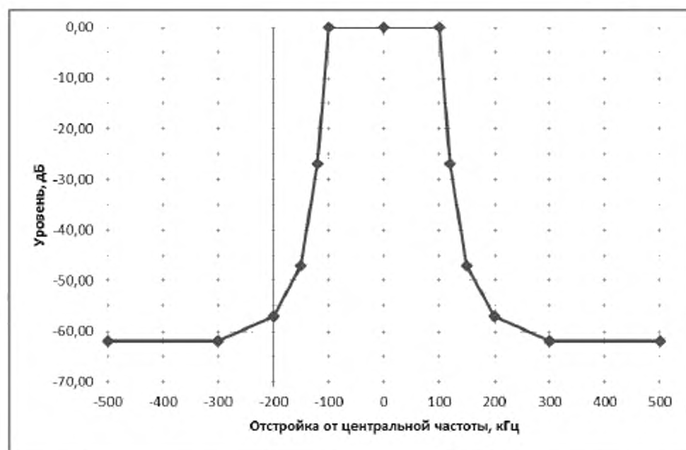
Рисунок А.2 – Маска огибающей внеполосных радиосигналов для условной ширины полосы частот 200 кГц
