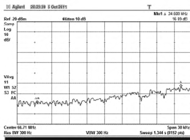
Рисунок В.20 – Форма спектра на частоте f_{(0-150)} в полосе сканирования 30 кГц
