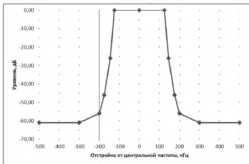
Рисунок А.3 – Маска огибающей внеполосных радиосигналов для условной ширины полосы частот 250 кГц
