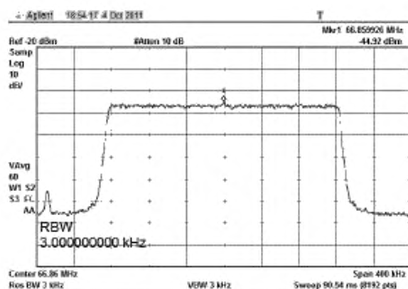
Рисунок В.35 – Полоса сканирования (Span) 400 кГц
