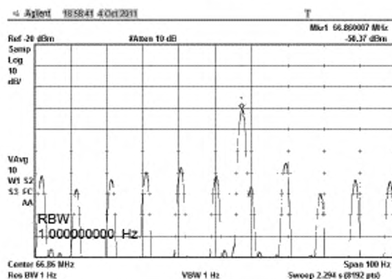
Рисунок В.39 – Полоса сканирования (Span) 100 Гц
