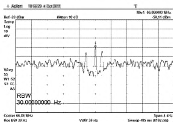
Рисунок В.37 – Полоса сканирования (Span) 4 кГц
