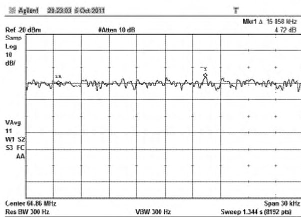
Рисунок В.18 – Форма спектра на частоте f_{(0)} в полосе сканирования 30 кГц
