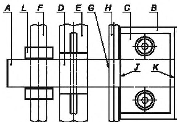
b) образец для испытания, сгибающий рычаг и направляющие ролики. вид сверху
