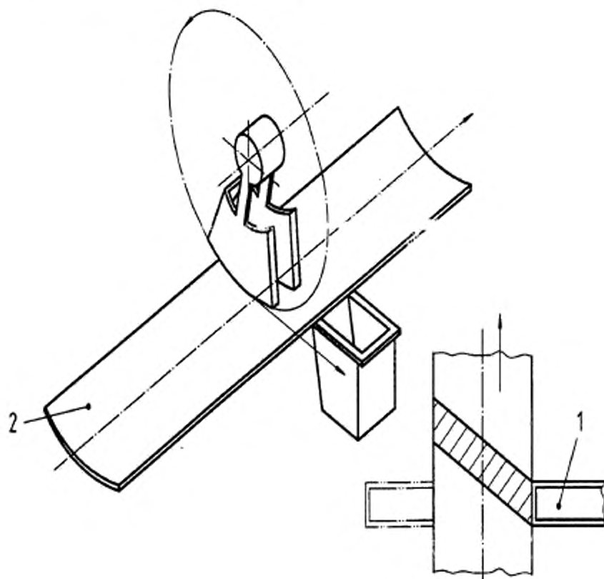
1 — отсекатель; 2 — лента конвейера с опорой для обеспечения ее кривизны
