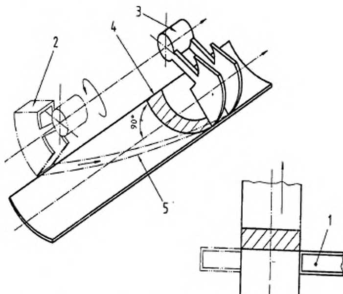
1—пробоотборник; 2—пробоотборник в нерабочей позиции; 3—пробоотборник в конце рабочего цикла; 4—поперечное сечение кокса, собираемого пробоотборником (и передаваемого в сборник); 5—траектория пробоотборника
