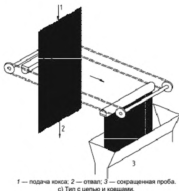
Рисунок 2, лист 3 — Примеры делителей
