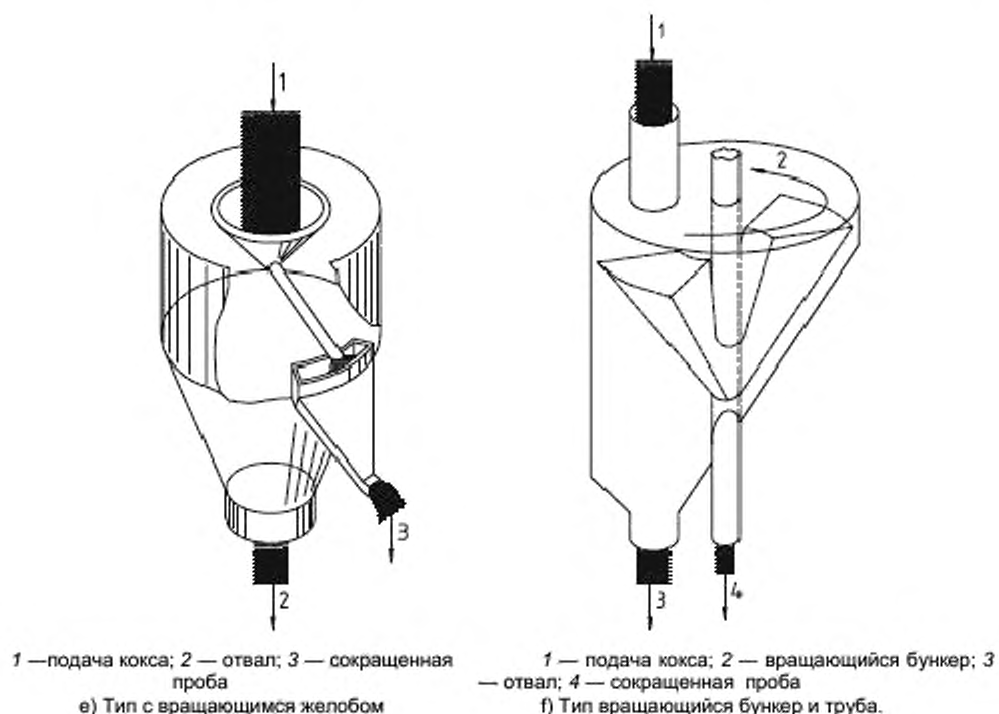
Рисунок 2, лист 5 — Примеры делителей
