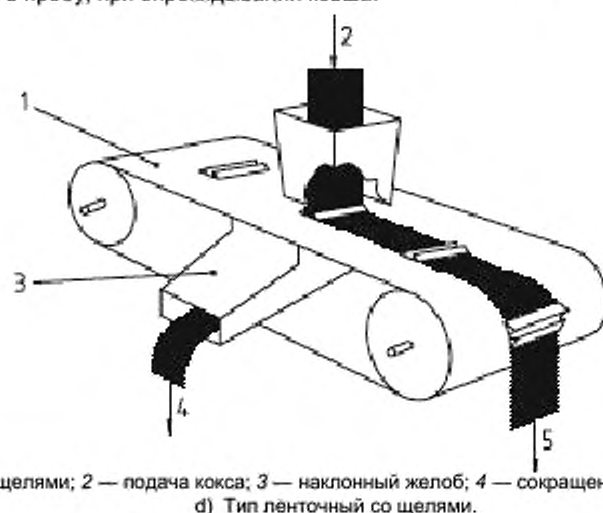
Рисунок 2, лист 4 — Примеры делителей
