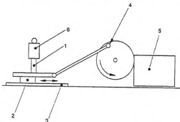
1 — слайд, 2 — войлочная прокладка, 3 — поверхность исследуемого образца, 4 — эксцентрик, 5 — электропривод, 6 — нагрузка
