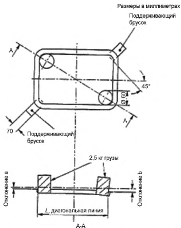
Рисунок Г.1 — Испытание на скручивание для подносов и блюдец
