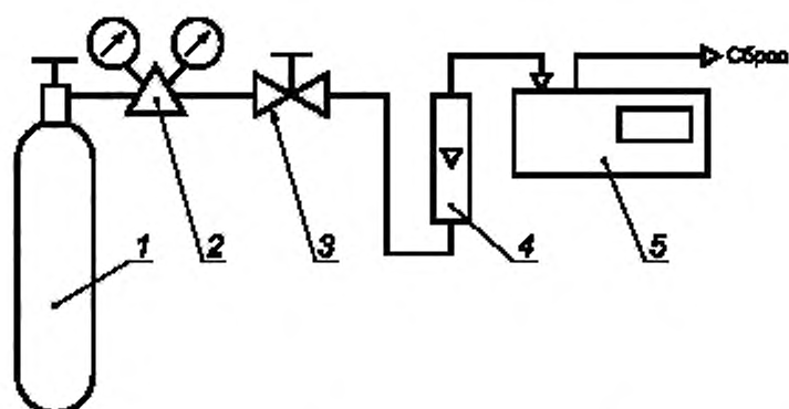
Рисунок Б.1 — Схема подачи ГС из баллонов под давлением на анализаторы, не оснащенные встроенным или внешним побудителем расхода
