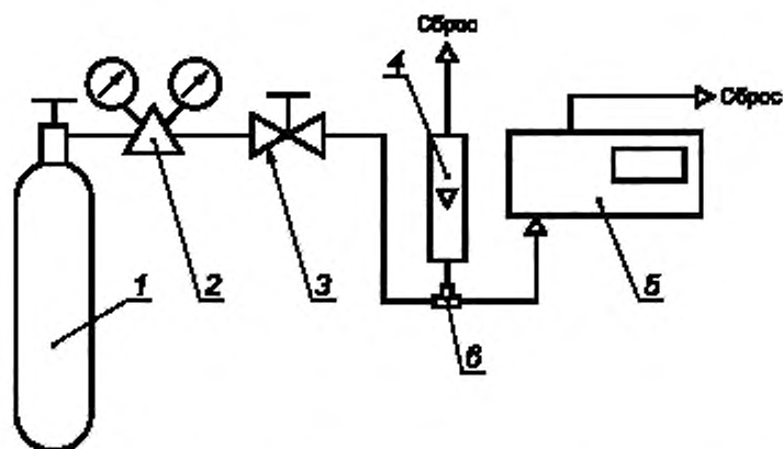
Рисунок Б.2 — Схема подачи ГС из баллонов под давлением на анализаторы, оснащенные встроенным или внешним побудителем расхода
