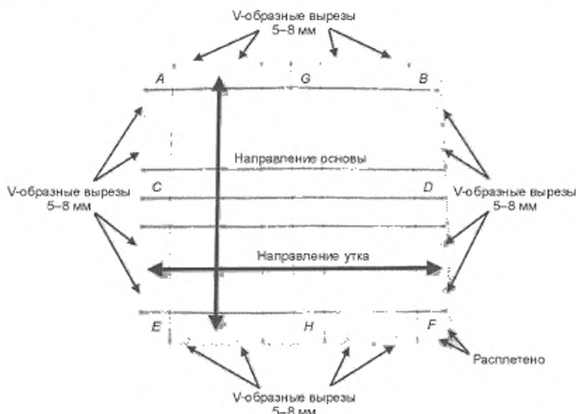
Рисунок 7 — Образец усадки шерсти, расплетенные кромки и V-образные вырезы
