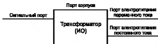
Рисунок 1 — Пример портов
