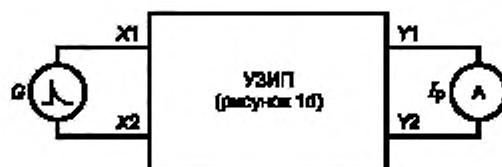
Рисунок E.4 — Определение сквозного тока дифференциального вида
