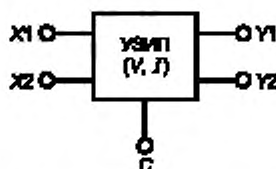
Рисунок 1е — Пятивыводное УЗИП
