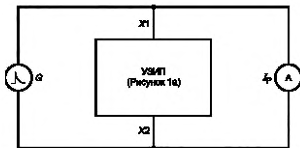
Рисунок Е.1 — Определение сквозного тока дифференциального вида
