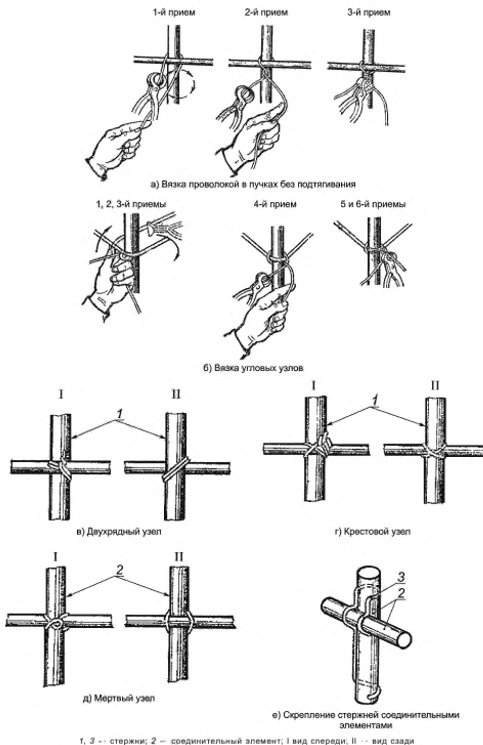
Рисунок Ж.2 – Приемы вязки проволокой пересечений арматурных стержней
