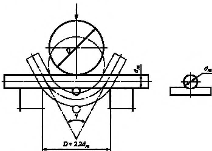
D — диаметр оправки; d_n — максимальный размер поперечного сечения испытываемого арматурного проката; \gamma — угол изгиба испытываемого арматурного проката
