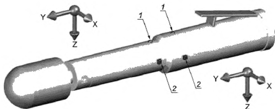
1 — предпочтительная точка измерений; 2 — дополнительная точка измерений
