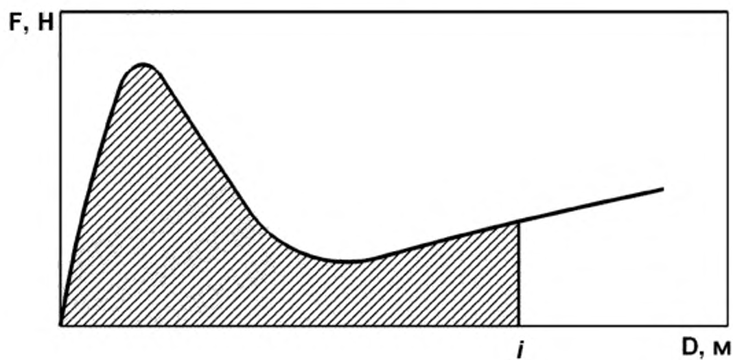
Рисунок А.1 – Зависимость силы от удлинения
