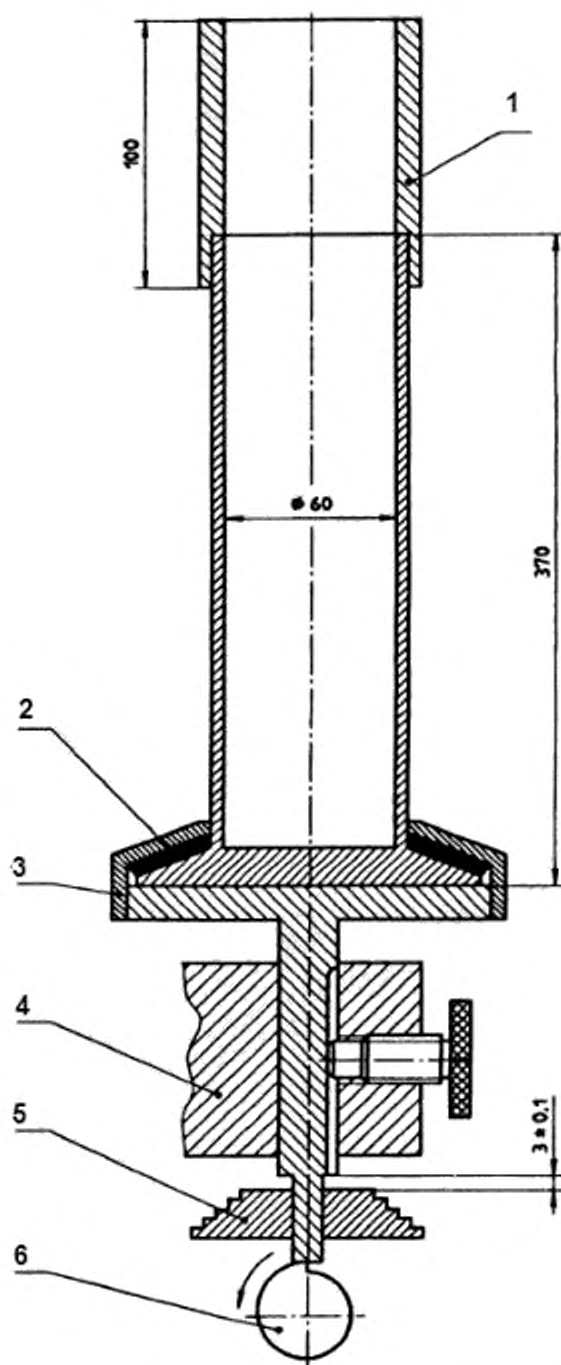
1 – кольцо; 2 – резиновое уплотнение; 3 – держатель измерительного цилиндра с направляющим зажимом; 4 – штучер; 5 – опора; 6 – кулачковый вал
