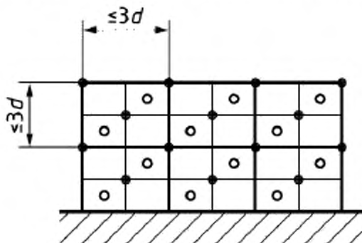
Рисунок С.1 – Основные точки установки микрофонов на измерительной поверхности в виде параллелепипеда с разбиением на прямоугольные участки
