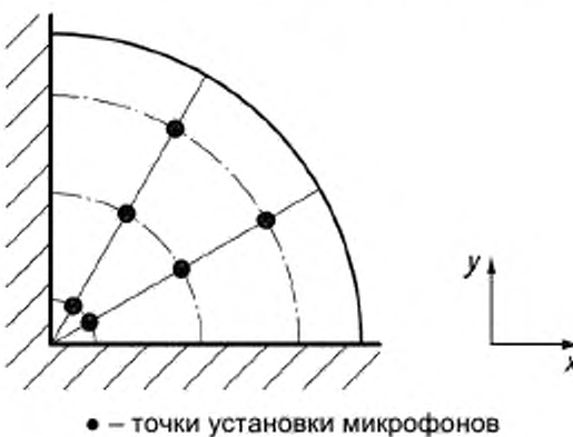
Рисунок D.4 – Пример расположения микрофонов на верхнем основании измерительной поверхности в виде четверти цилиндра в случае трех звукоотражающих плоскостей
