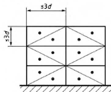
Рисунок С.3 – Пример дополнительных точек измерений на части измерительной поверхности в виде параллелепипеда с разбиением на прямоугольные участки
