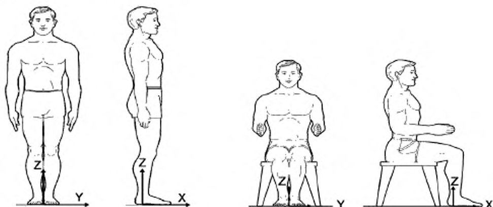
Рисунок 1 — Оси координат x , y , z .
