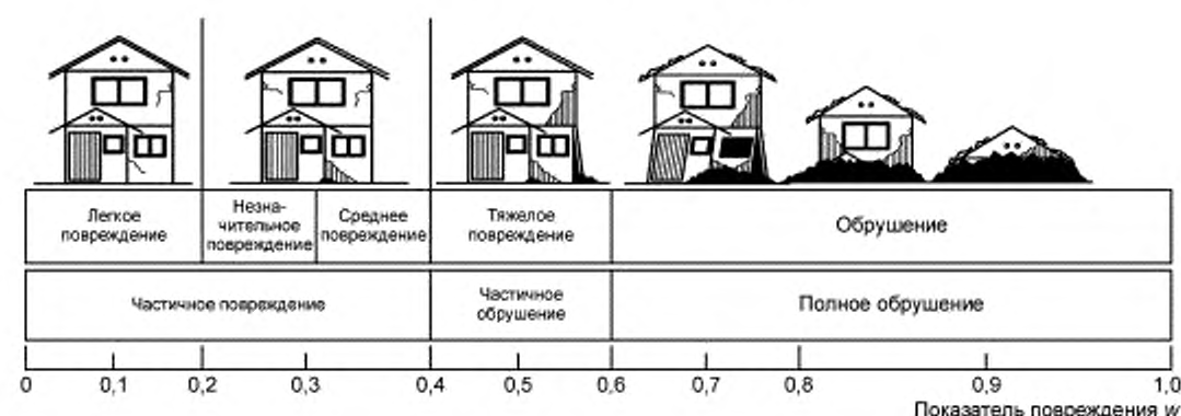
Рисунок Н.1 — Степень и показатель повреждения
