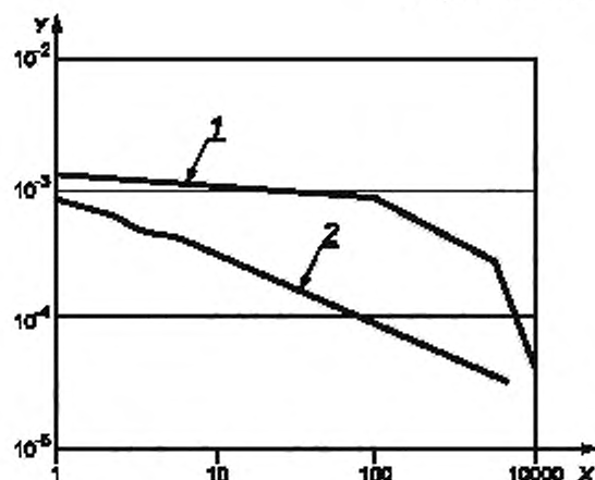
Рисунок D.1 — Пример кривых риска
