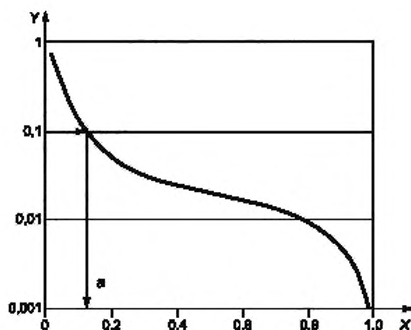
Рисунок D.4 — Взаимосвязь между кривой риска и МВУ
