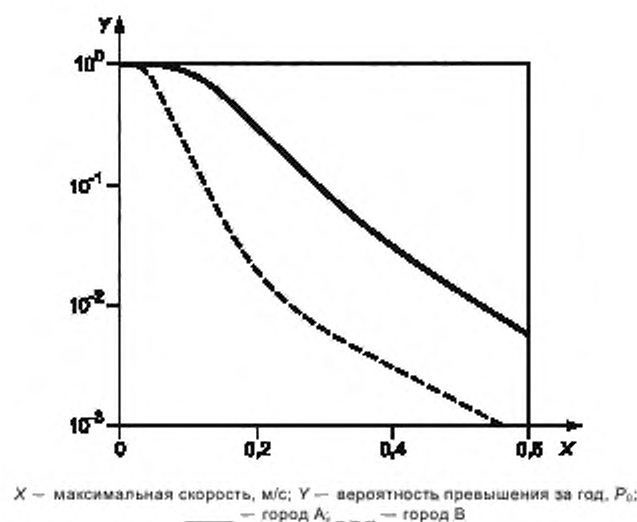
Рисунок Е.1 — Пример кривой сейсмического риска
