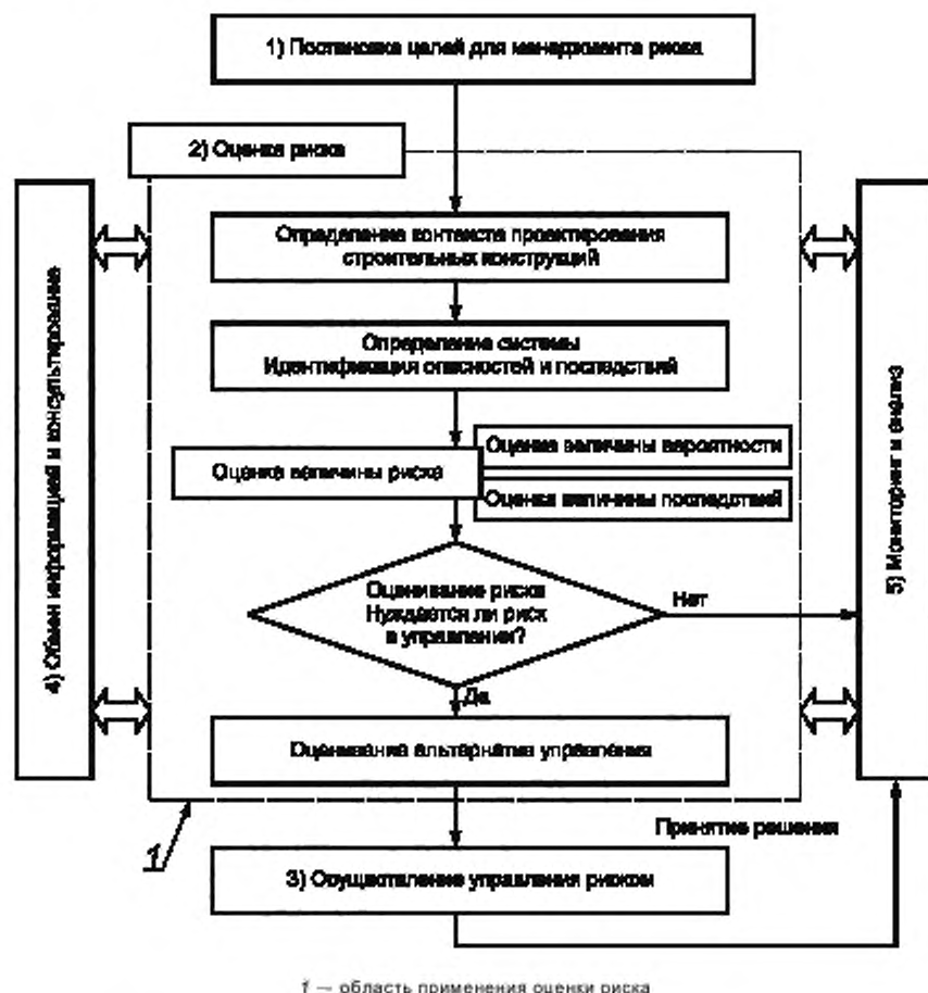
Рисунок 1 — Процесс менеджмента риска и область применения оценки риска для систем, включающих строительные конструкции
