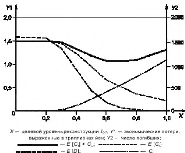
Рисунок Н.2 — Целевой уровень и ожидаемые потери
