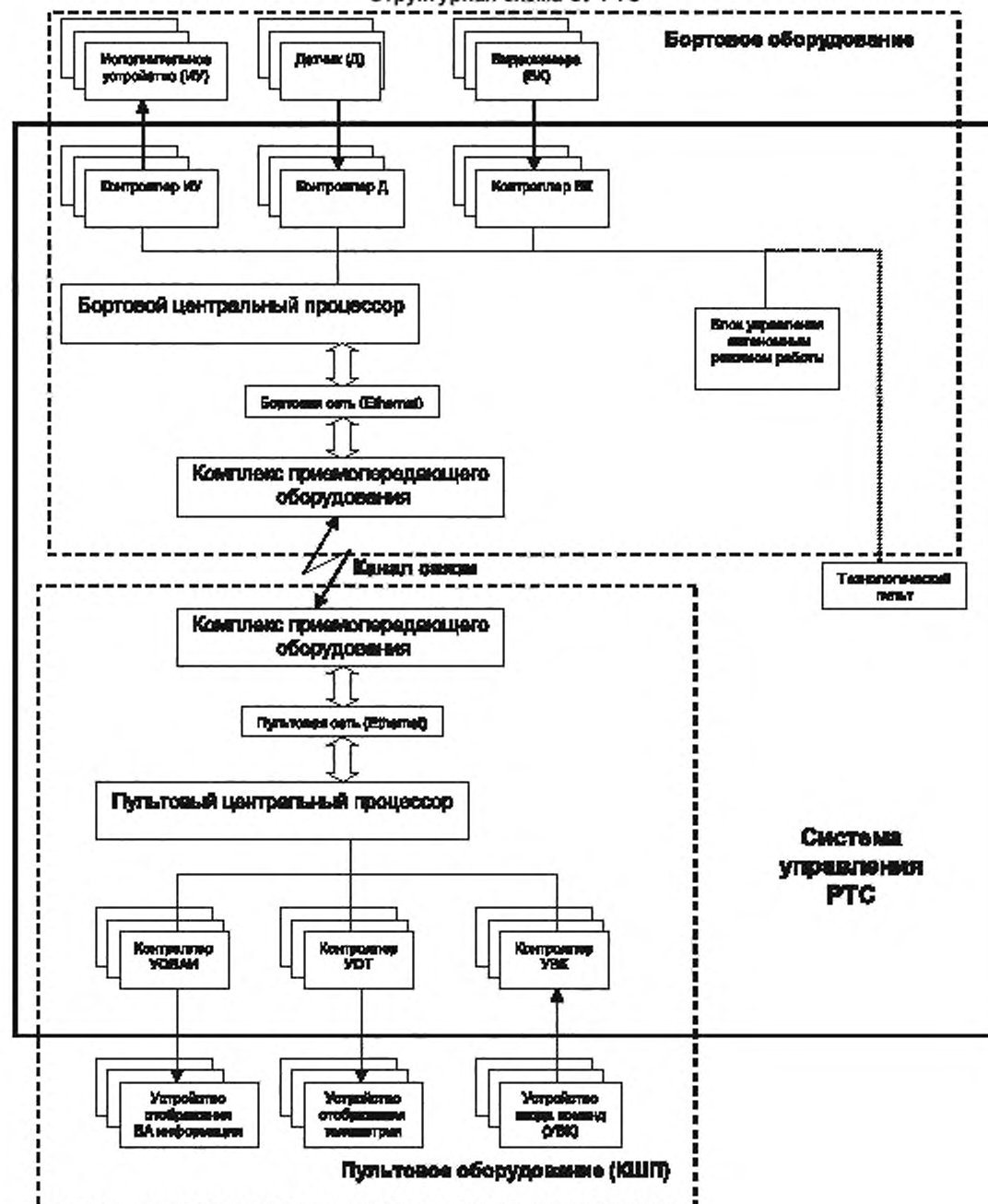
Структурная схема СУ РТС
