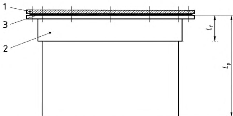
1 – металлический фланец; 2 – фиксированный фланец из стеклокомпозита; 3 – уплотнитель; L_f – длина фланца; L_t – длина трубы
