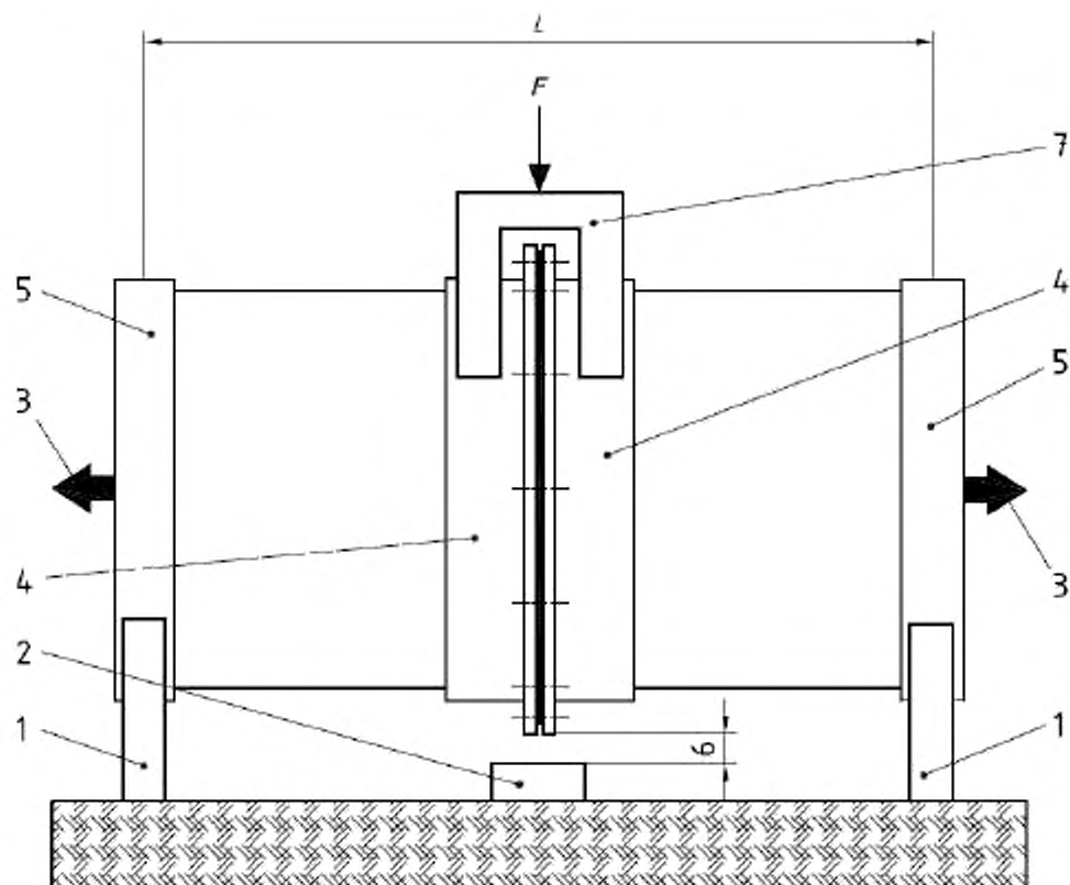
1 — опора; 2 — ограничитель; 3 — осевая нагрузка, действующая на образец; 4 — испытуемые стеклокомпозитные фланцы; 5 — жесткие заглушки; 6 — предельное отклонение соединения в середине пролета; 7 — лотковая опора, передающая изгибающую нагрузку; L — длина; F — дополнительная изгибающая сила (при необходимости)
