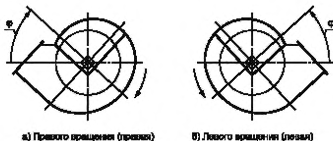
Рисунок 3 — Центробежные ТДМ правого и левого вращений
