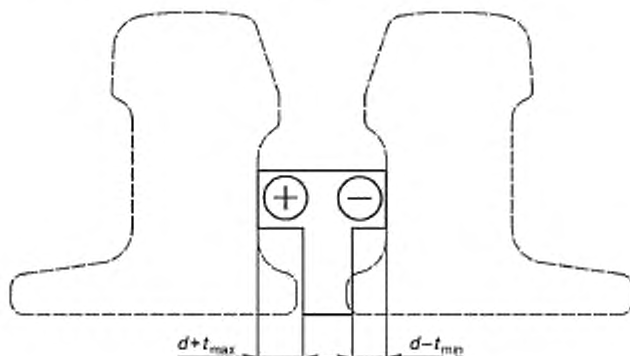
Рисунок Е.6 — Шаблон контроля толщины шейки рельса
