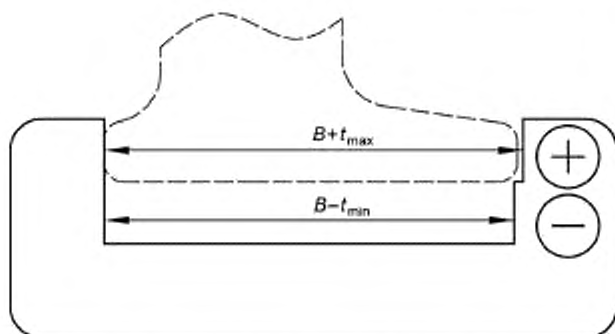
Рисунок Е.5 — Шаблон контроля ширины подошвы рельса
