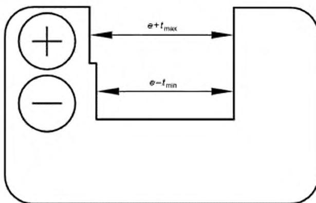
Рисунок Е.5 — Шаблон контроля ширины подошвы рельса
