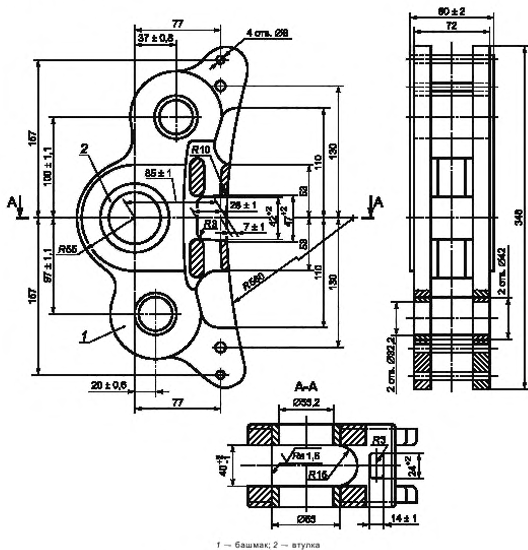
Рисунок 5 — Башмак типа 2 — Исполнение 1
