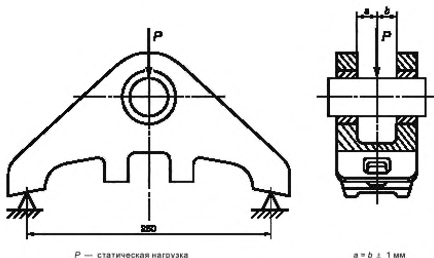
Рисунок В.1 — Схема испытания башмака статической нагрузкой
