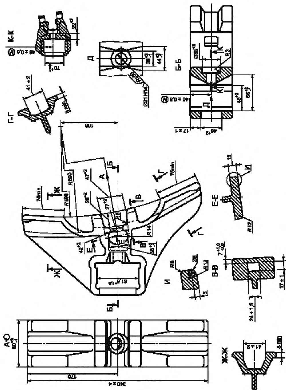
Рисунок 2 — Башмак — тип 1/Исполнение 1
