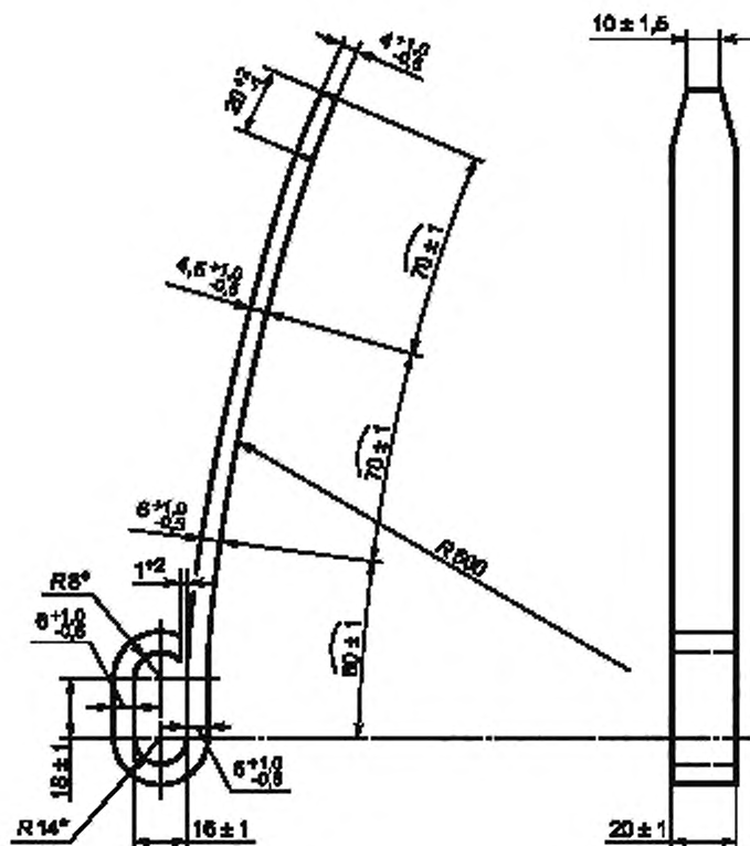
Рисунок 14 — Чека типа 4
