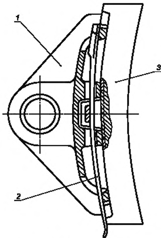
1 — башмак; 2 — чека; 3 — колодка
