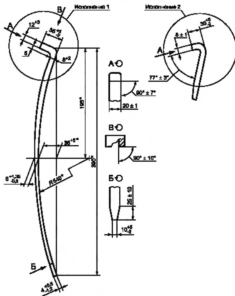
Рисунок 11 — Чека типа 1
