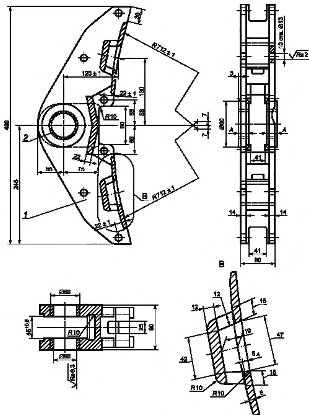
Рисунок 9 — Башмак секционный типа 4
