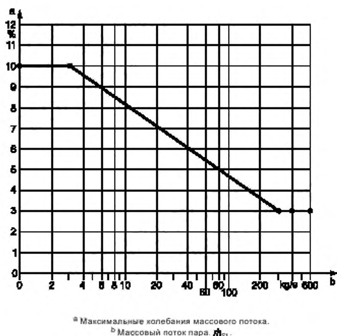
Рисунок 6.6-1 — Максимально допустимые колебания массового потока пара
