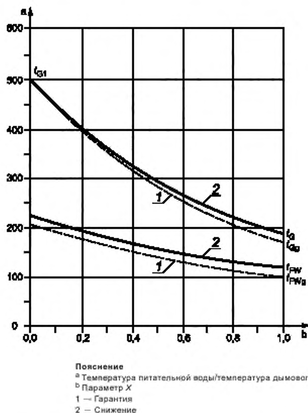
Рисунок 9.5-1 — Изменение температуры в подогревателе питательной воды (X — любой параметр)
