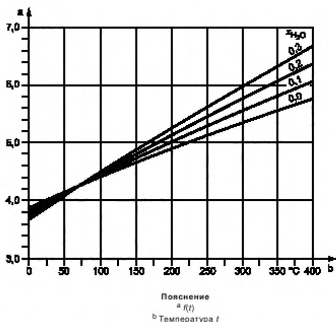
Рисунок 10.4-1 — Функция для расчета коэффициента теплопередачи по линии
