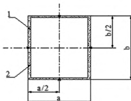
1 — воздухопровод; 2 — покрытие воздухопровода; • — ТЭП; a , b — размеры поперечного сечения воздухопровода
