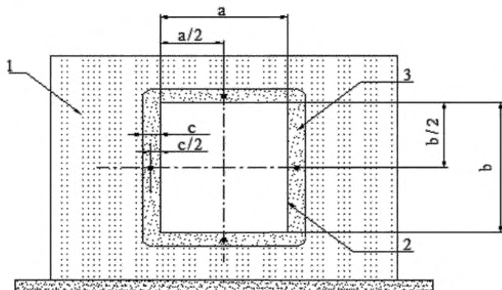
1 — печь; 2 — воздухопровод; 3 — уплотнение места прокладки воздухопровода через ограждающую конструкцию печи; • — ТЭП; a , b — внутренние размеры поперечного сечения воздухопровода; c — толщина заделки
