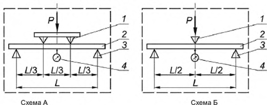
Рисунок 1 – Схема установки для определения модуля упругости
