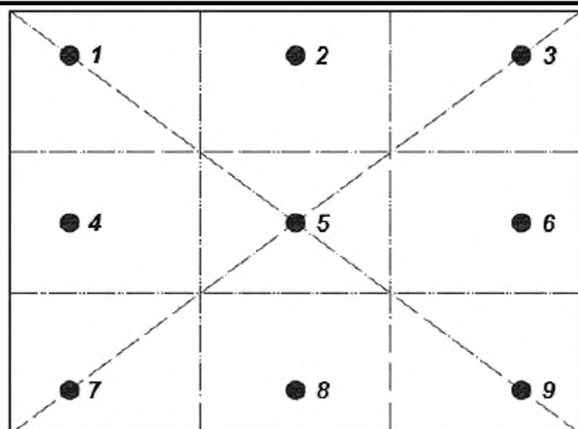
Рисунок 12 – Расположение точек измерений на анизотропном излучающем плоскостном ЖК-дисплее (преобладает реальная информация)
