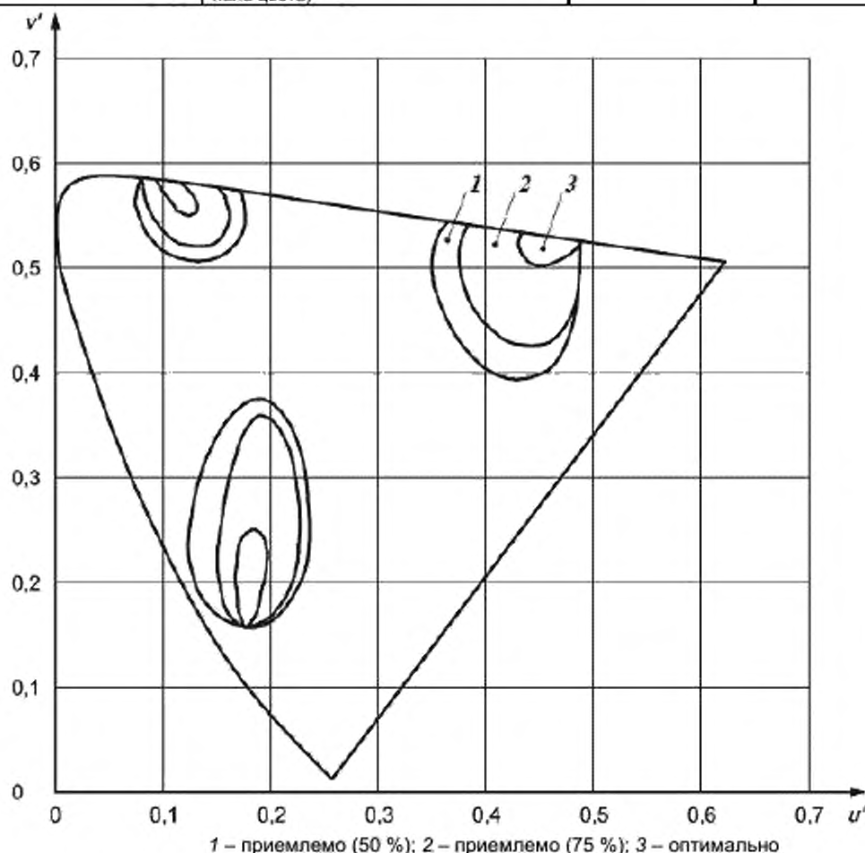
Рисунок 16 – Оптимальный и приемлемый цветовые диапазоны. Плазменные дисплеи
