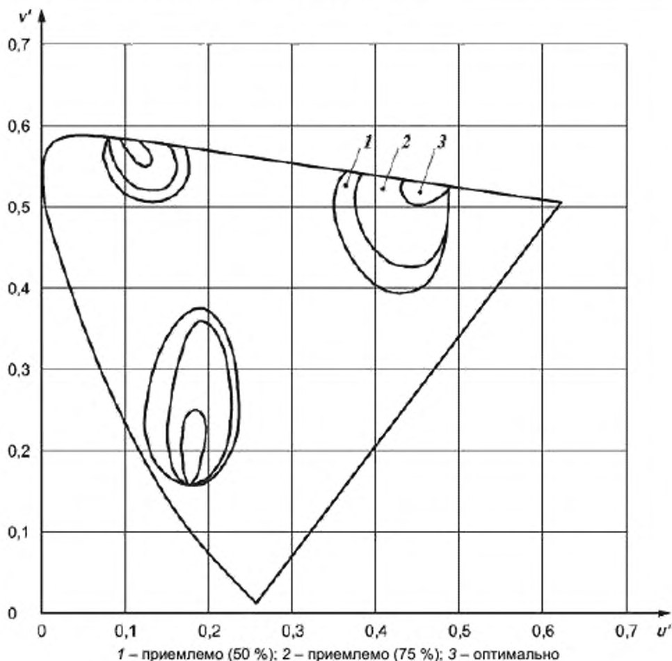
Рисунок 4 – Оптимальный и приемлемый цветовые диапазоны. ЭЛТ-дисплеи
