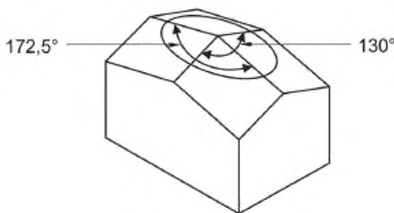
Рисунок 2 – Индентор Кнупа
