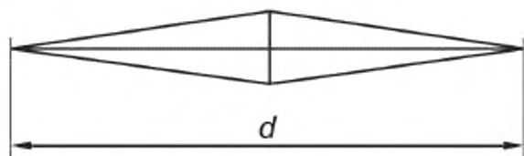
Рисунок 1 — Проекция отпечатка, полученного с помощью индентора Кнупа
