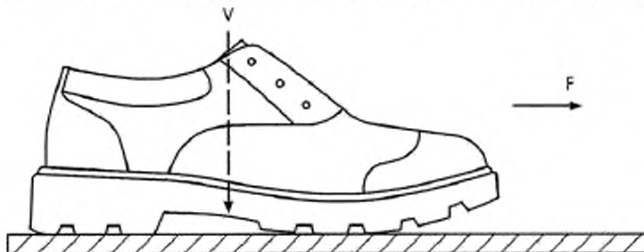
в) Режим плоского скольжения вперед при использовании механической ноги или колодки изготовителя V — нормальная сила; F — движение обуви относительно поверхности; B — обратное движение обуви относительно поверхности
