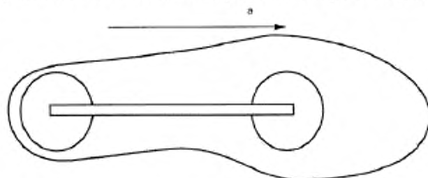
Рисунок 3 — Продольная ось механической ноги параллельная направлению движения
