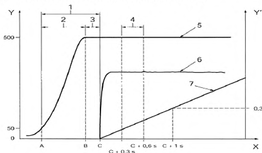
Рисунок 4 — Иллюстрация графика испытания при нормальной силе 500 Н
