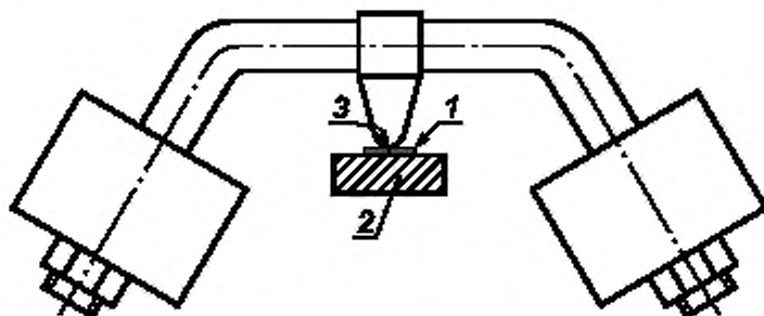
1 — образец; 2 — опора; 3 — сферический радиус R = 2,5 мм
