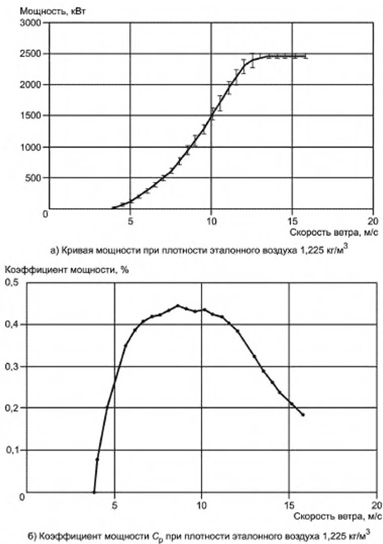
Рисунок 4 — Пример выборочных данных: кривая измеренной мощности и кривая C_p
