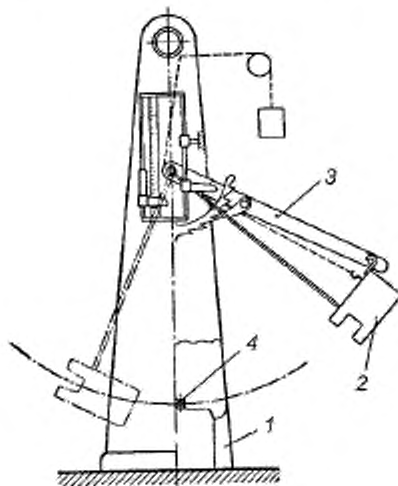
1 - стойка; 2 - маятник; 3 - подъемная рама; 4 - образец
