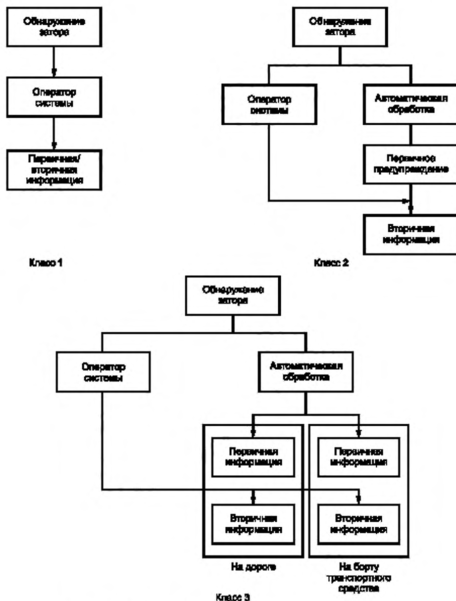
Рисунок 2 — Процессы обеспечения информацией для каждого класса
