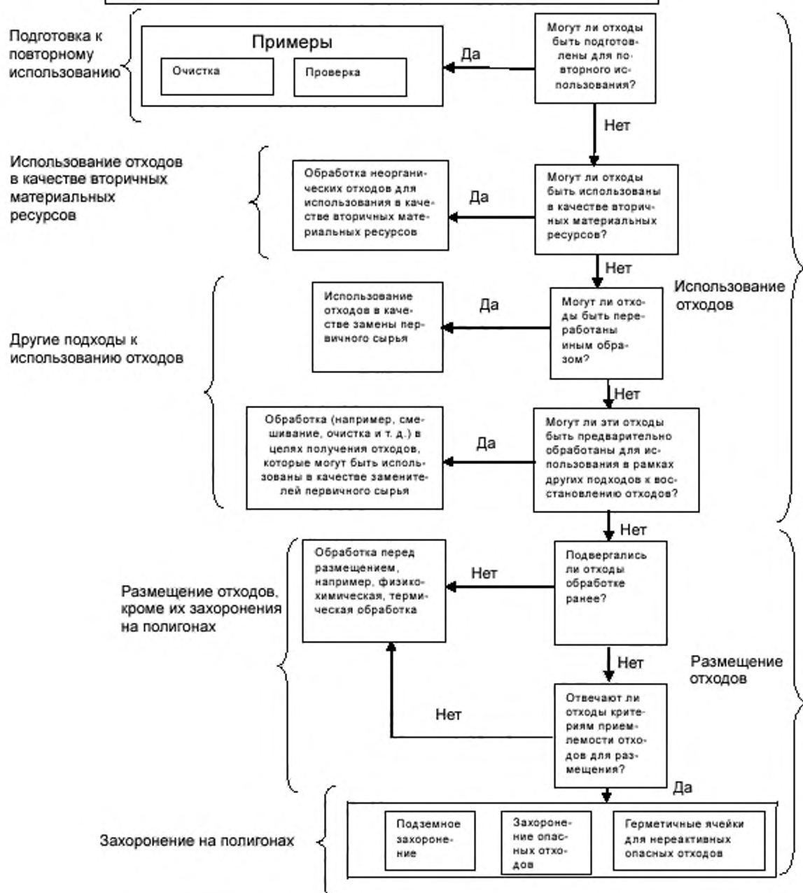
Рисунок Б.5.1 — Порядок принятия решений при обращении с неорганическими отходами
