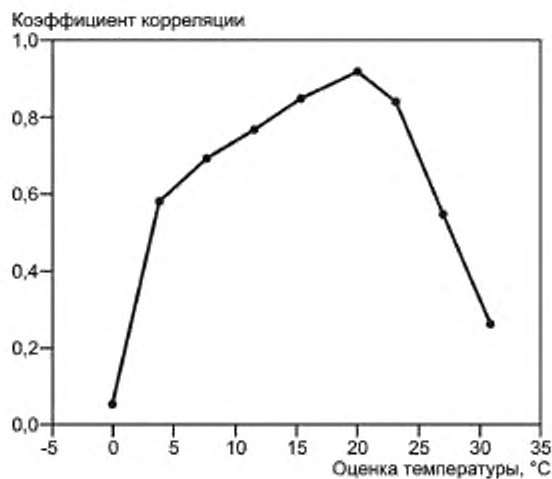
Рисунок 23 — Коэффициент корреляции, соответствующий паре оценок \hat{\theta}_j и \hat{\theta}_{10} температур \theta_j и \theta_{10} = 20\text{ °C} (9.5.3.7)
