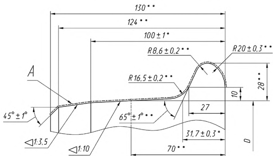
Профиль колеса с толщиной гребня 27 мм
