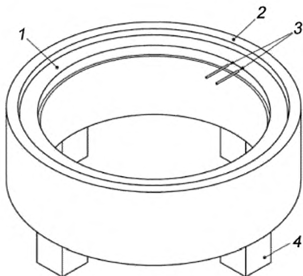
1 — металлическое кольцо; 2 — держатель основы; 3 — металлические стержни; 4 — опоры
