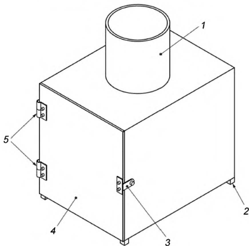
Рисунок А.1 — Общий вид испытательной камеры
