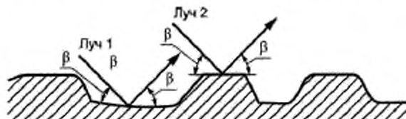
Рисунок D.1 — Критерий неровности поверхности пластины заземления (по Релею)
