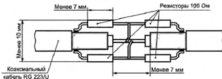
Рисунок С.3 — Конструкция антенной прорези
