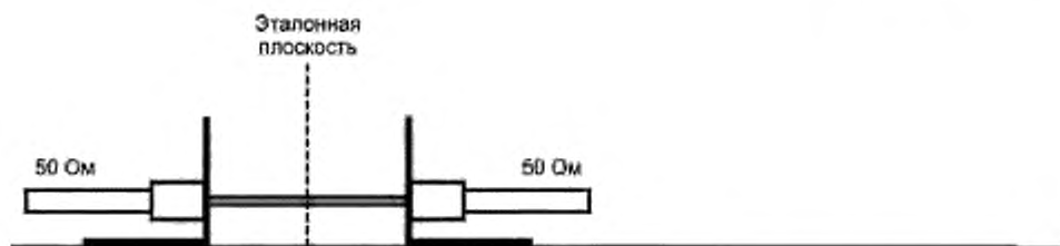
Рисунок 24с) — Конфигурация при калибровочном измерении «Насквозь»
