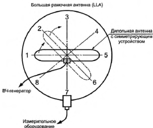
Рисунок С.7 — Восемь положений установки диполя при валидации большой рамочной антенны
