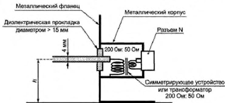
Рисунок 26 — Пример конструкции адаптера 50 Ом в вертикальном фланце зажимного устройства
