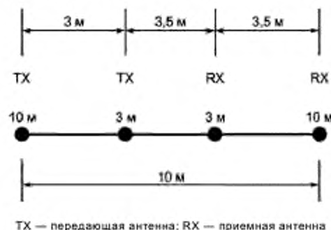
Рисунок 31 — Размещение испытательных точек для измерительного расстояния 3 м
