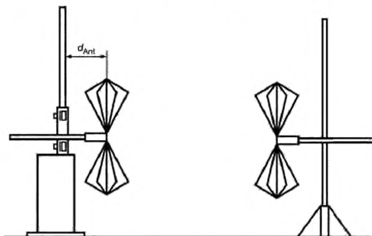
Рисунок 34 — Пример анализа влияния мачты антенны на AAPR
