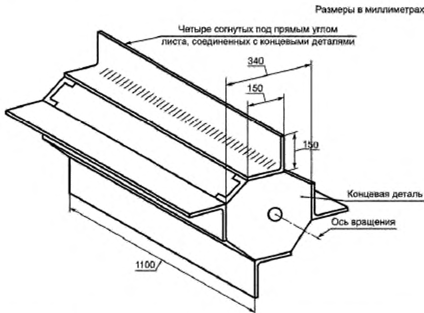
Рисунок 16 — Пример типичного рассеивающего устройства с вращающимися лопатками
