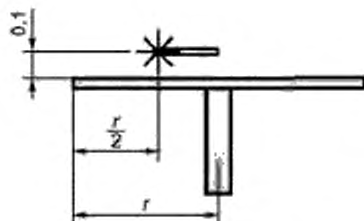
Рисунок 15 — Позиция антенны над установочным столом (вид сбоку)
