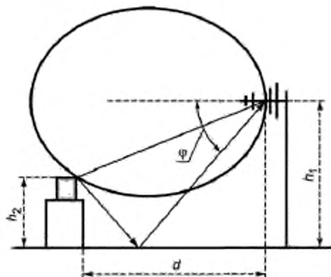
Рисунок 1 — Схема излучения от ТС, попадающего на антенну LPDA напрямую и за счет отражения от земли, на площадке с расстоянием 3 м, демонстрирующая половину ширины диаграммы направленности \varphi , при отраженном луче
