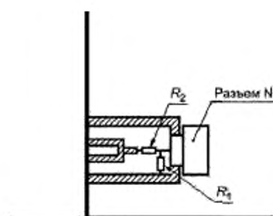
Рисунок 28 — Пример согласующего адаптера с резистивной схемой согласования
