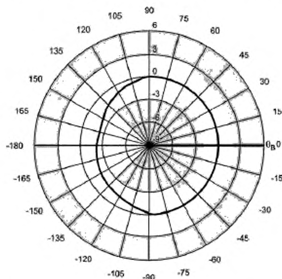
Рисунок 19a) — Диаграмма излучения передающей антенны в плоскости H на частотах от 1 до 6 ГГц
