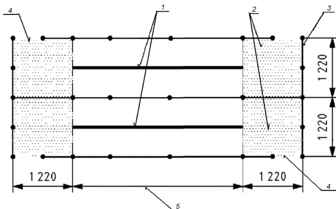
б) Параллельное размещение подвесных дорог
