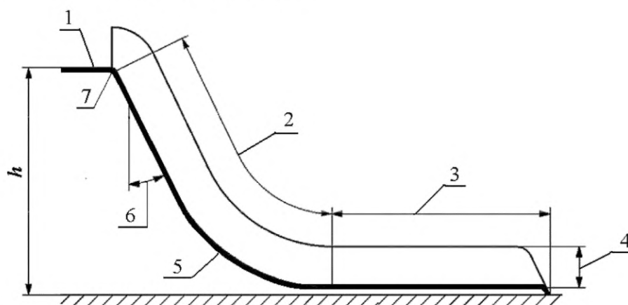
1 — стартовый участок; 2 — участок скольжения; 3 — конечный участок; 4 — бортики; 5 — радиусный элемент нижней части участка скольжения; 6 — угол наклона участка скольжения к вертикали; 7 — радиусный элемент верхней части участка скольжения (не менее 100 мм); h — высота горки
