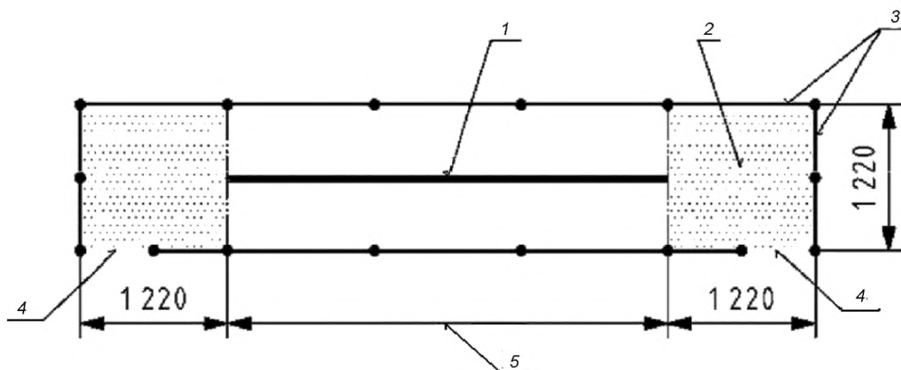
а) Одиночная подвесная дорога
