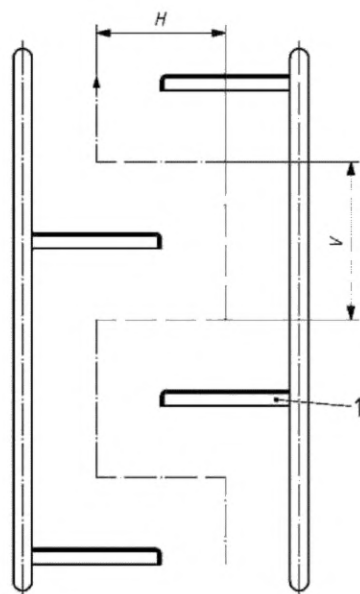
1 — платформа; H — горизонтальное расстояние; V — вертикальное расстояние
