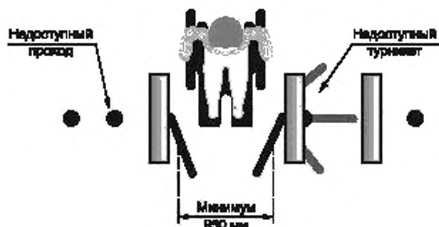
Рисунок 8 — Проход через турникет
