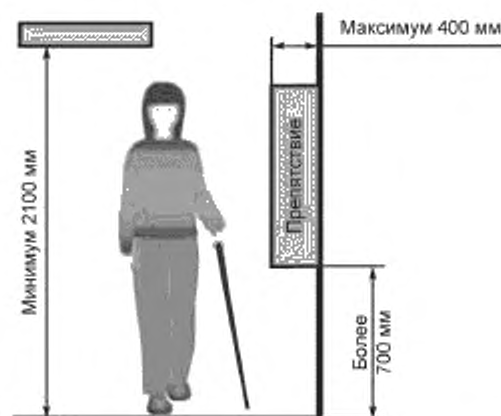
Рисунок 2 — Предельные размеры выступающих объектов
